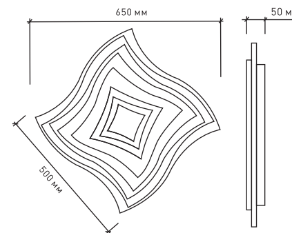
GEOMETRIA QUADRATE 85W Q
